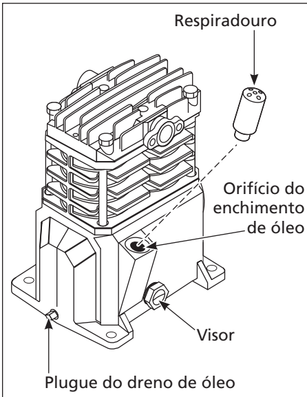
Figura 2 - Abastecer Óleo
