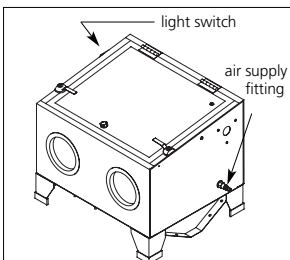
Figura 3 - Cabina de chorreado de mesa
