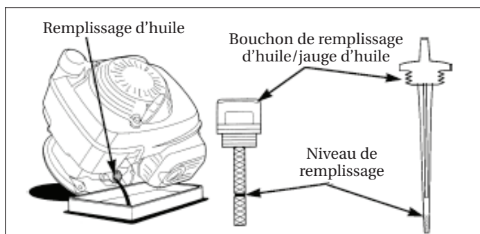
Figure 20 - Vidange d'huile et endroit pour le remplissage d'huile
