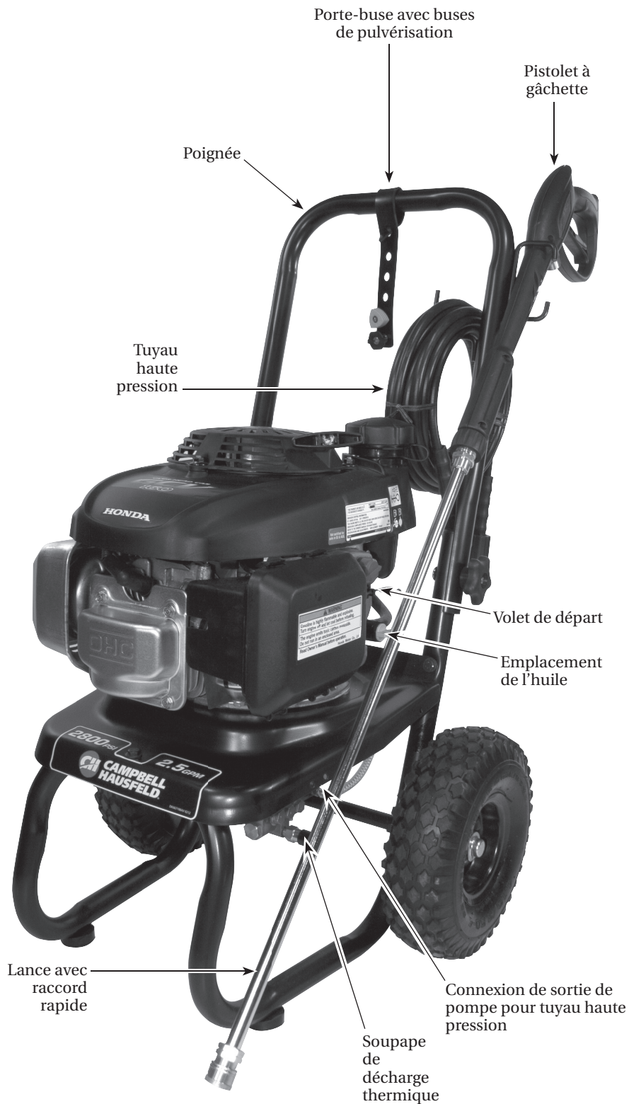
Figure 7 - Composants de la laveuse à pression
