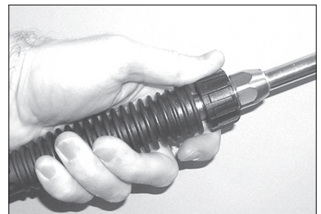
Figura 11 - Conecte la lanza a la pistola
