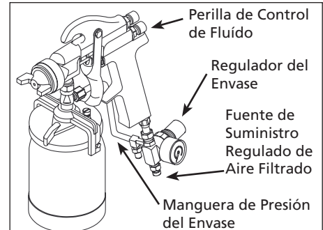
Figura 3 - Conexión del Sistema a Presión
