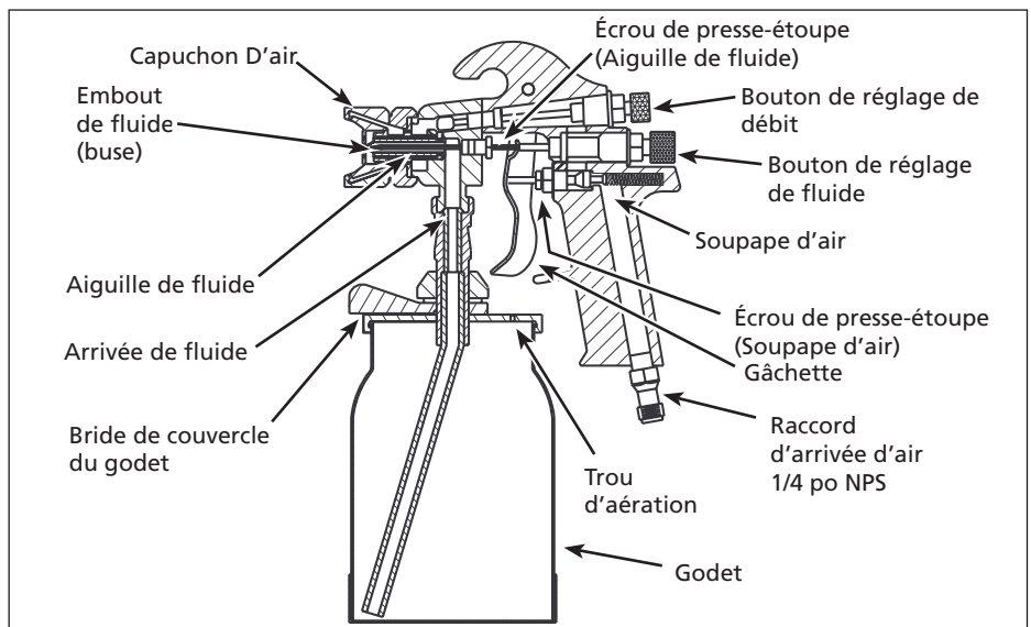
Figure 14 - Pistolet Vaporisateur Conventionnel À Siphon
