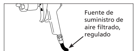
Figura 5 - Conexión del sistema de gravedad
