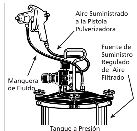
Figura 4 - Conexión del Tanque a Presión
