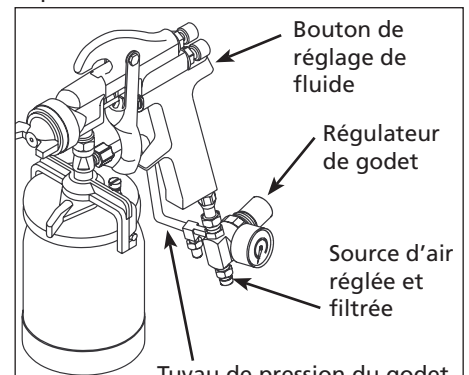
Figure 3 - Montage du Godet pour Alimentation Sous Pression
