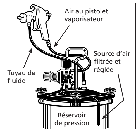
Figure 4 - Montage du réservoir pour l'alimentation sous pression
