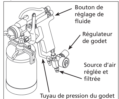
Figure 3 - Montage du Godet pour Alimentation Sous Pression
