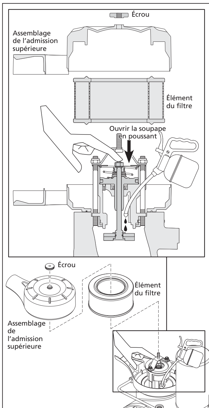
Figure 9 - Emplacement d'amorçage de l'extrémité d'air
