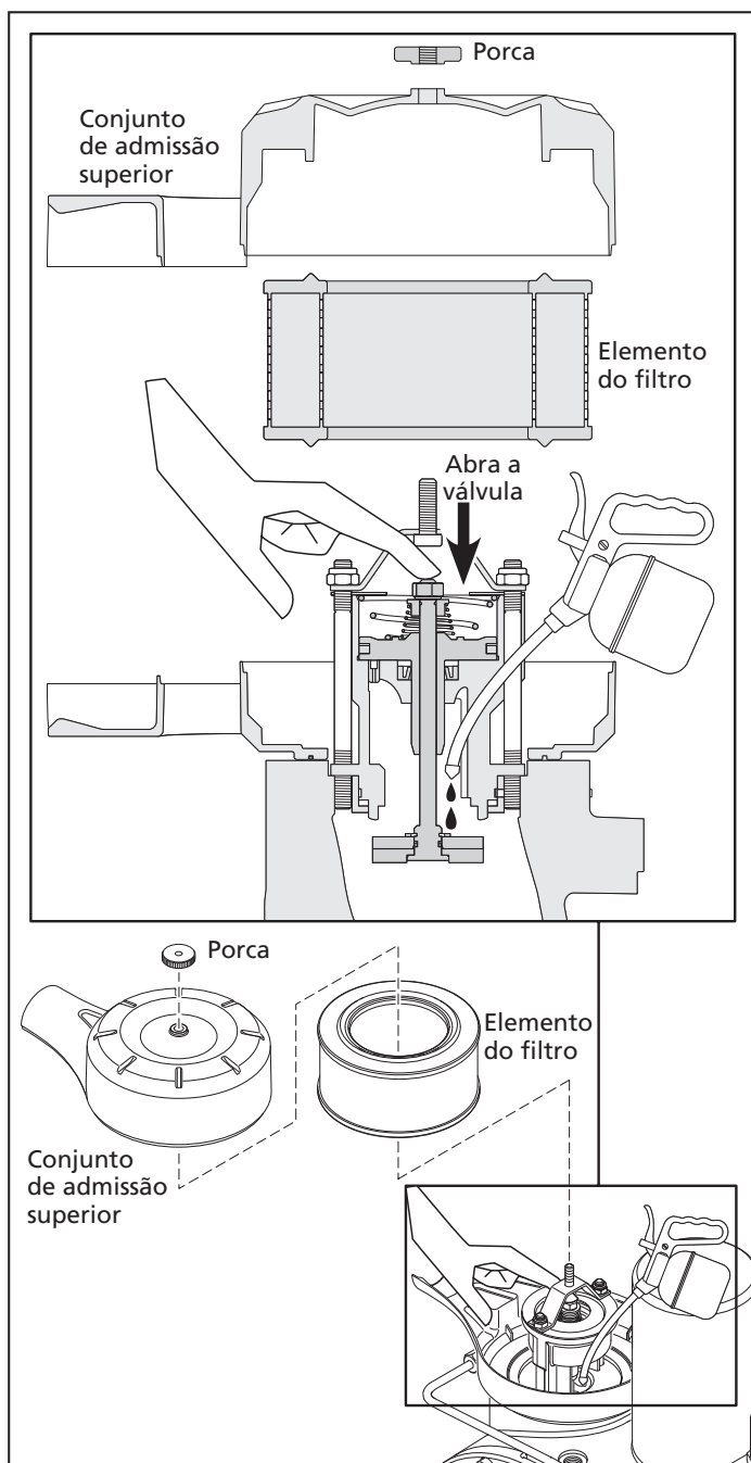
Figura 9 - Local de escorva de extremidade de ar
