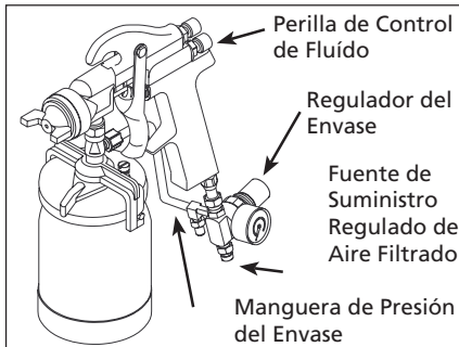
Figura 3 - Conexión del Sistema a Presión
