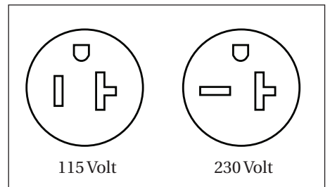
Figura 4 – Tomacorriente
