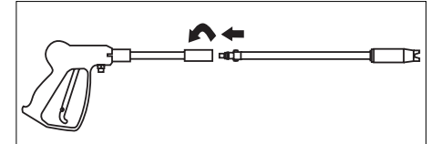
Figura 4 - Conexión de la pistola y lanza
