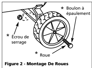
Figure 2 - Montage De Roues
