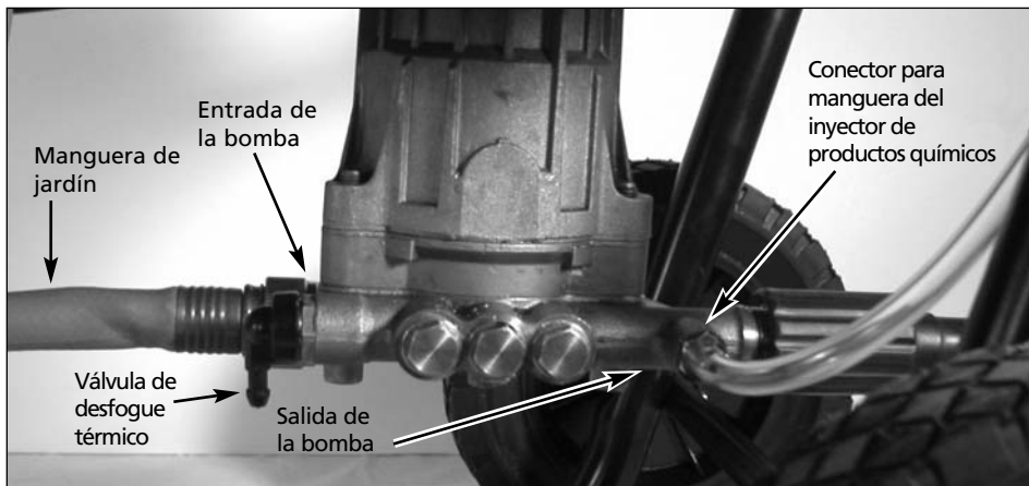
Figura 2 - Conexión de la bomba
